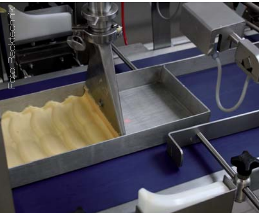
Bild links: Die Hebe-Senk-Düse ist auf die Breite des Bleches abgestimmt und füllt die Masse sehr gleichmäßig in die Form ein. Bild Mitte: Abteilungsleiter Jens Dose (links) und Thomas Dreler sind für die Abläufe an der Dosieranlage zuständig. Bild rechts: Die Masse hat sich schnell und gleichmäßig auf dem Blech verteilt, so dass ein weiteres Verstreichen entfällt und sofort mit dem Belegen begonnen werden kann.
